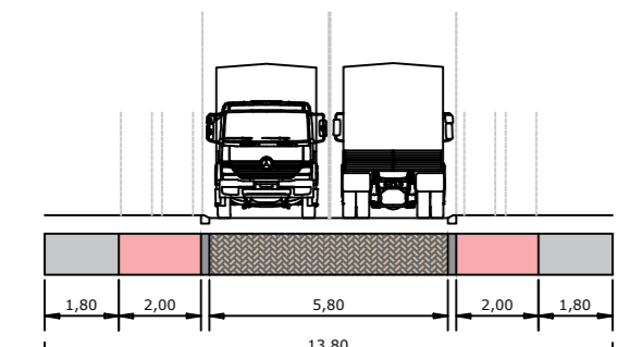
Profiel GOW30 tot 10.000mvt
