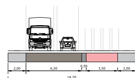
Profiel éénrichtingsverkeer met opstelruimte
