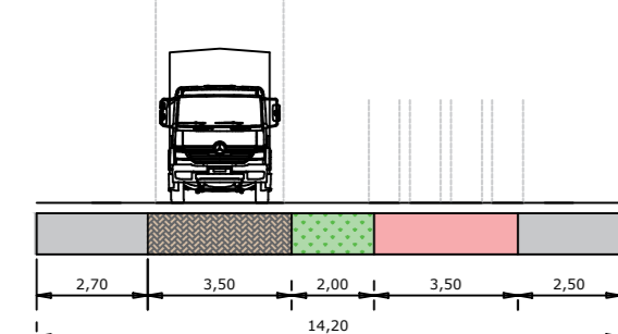
Profiel GOW30 tot 10.000mvt
