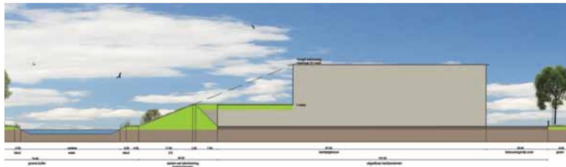
verschillende mogelijkheden overgang dijklichaam - bedrijfsbebouwing
