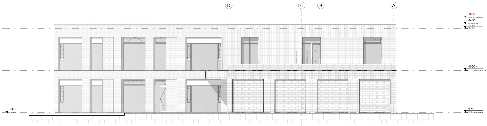
gevel - west
