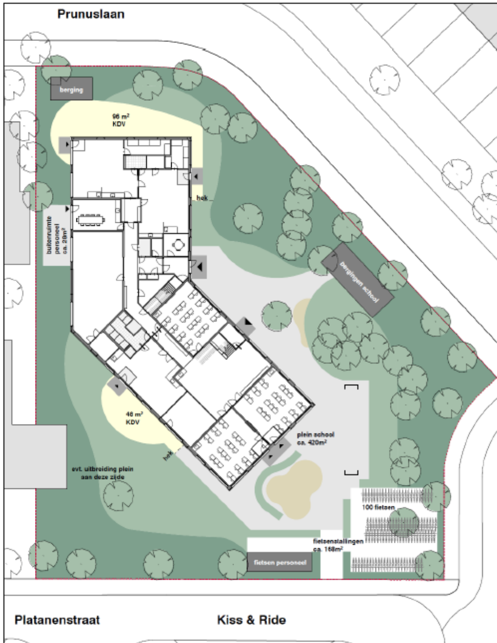
Figuur 1 Situatiekening
