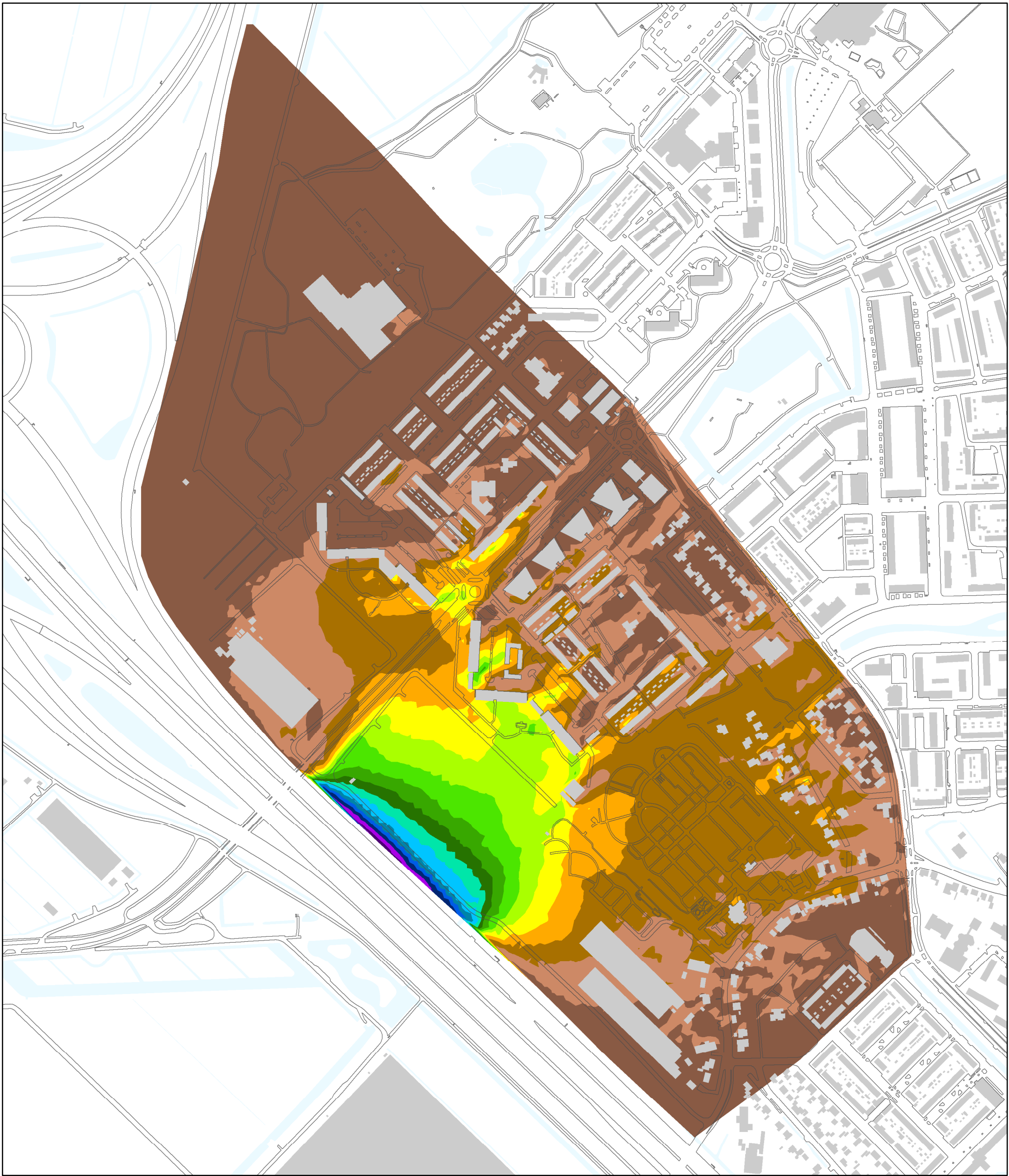
Verschilcontouren bestaande situatie versus geluidscherm 6 meter
